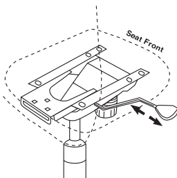
Knee tilt - KNT2
