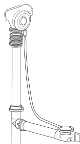
# 791264 (plástico) # 790250 (metal) La versión Cape Cod incluye un desagüe instalado de fábrica.
