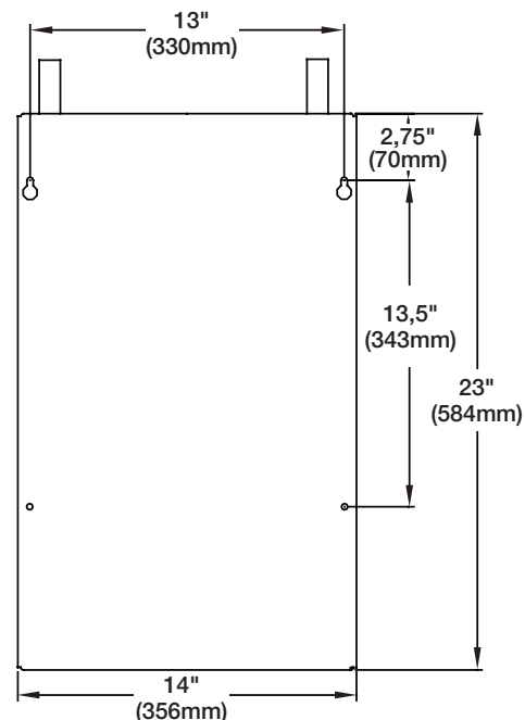
Vue de côté - Trous de fixation murale (NEMA 1)
