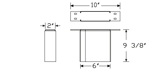
credenza stanchion
