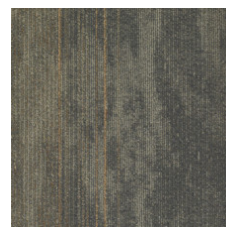
Hematite 14760
