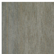
Galena 14515
