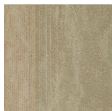
Gypsum 14111
