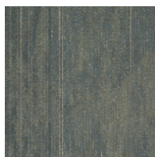
Azurite 14315
