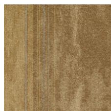
Amber 14200
