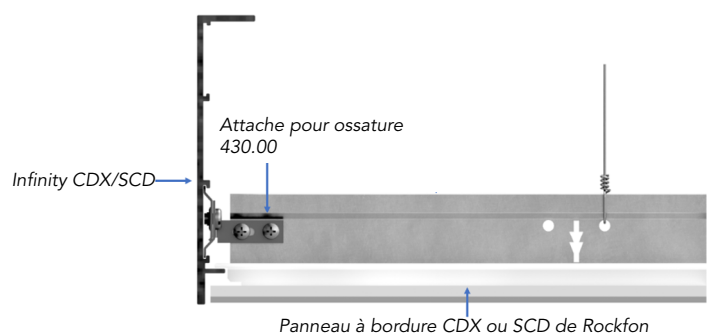
Installation d'Infinity CDX sur une ossature avec panneau à bordure CDX de Rockfon
