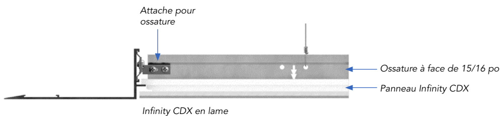
Installation d'Infinity CDX en lame sur une ossature avec panneau à bordure CDX de Rockfon
