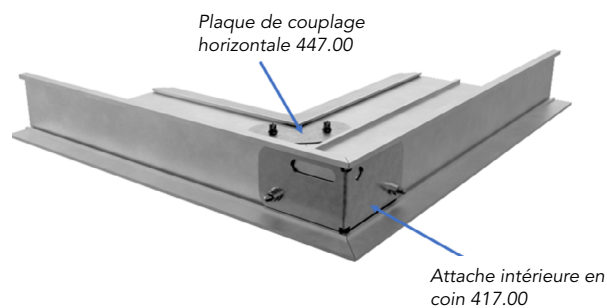
Installation de coin intérieur
