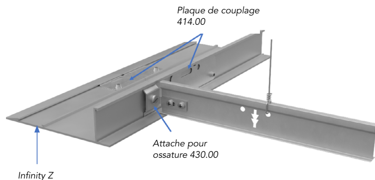
Installation d'Infinity Z sur une ossature de plafond suspendu
