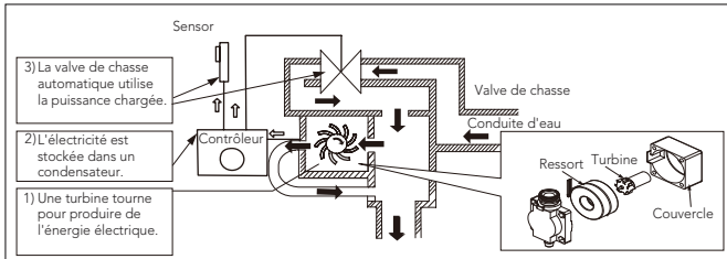
fig. 1 Générateur Hydropowered
