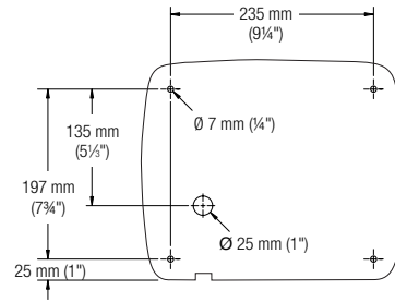
Plantilla de montaje, vista delantera
