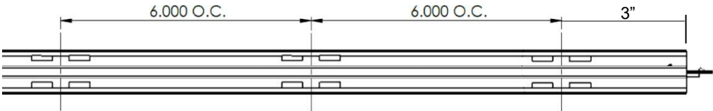
Flange Slots for EZTS
