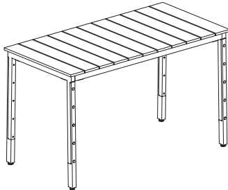
36" Counter Height Rectangle OSPBA2436 OSPBA3036 OSPBA3642 OSPBA2442 OSPBA3042 OSPBA3648 OSPBA2448 OSPBA3048 OSPBA3654 OSPBA2454 OSPBA3054 OSPBA3660 OSPBA2460 OSPBA3060 OSPBA3666 OSPBA2466 OSPBA3066 OSPBA3672 OSPBA2472 OSPBA3072 OSPBA3684 OSPBA2484 OSPBA3084 OSPBA3696 OSPBA2496 OSPBA3096
