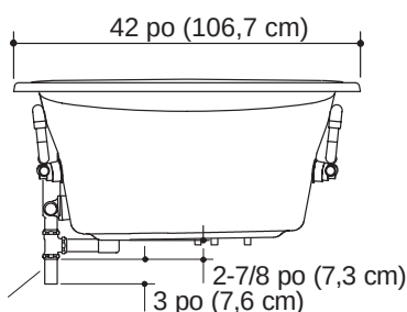
DÉTAIL DE REBORD POUR INSTALLATIONS SURBAISSÉES
