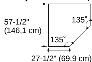
Detalle de la abertura de los modelos con borde empotrado
