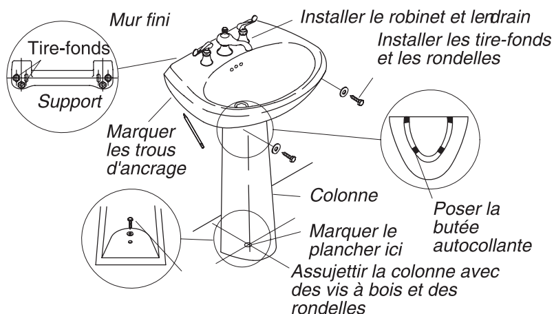
Emplacement de la colonne et du lavabo
