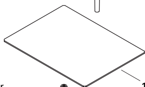
1059111** Cadre inférieur
