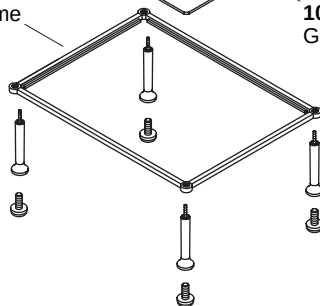
1058920** Foot
